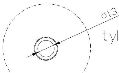
WIDOK W WERSJI BEZ BAJONETU VIEW WITHOUT BAJONET SOCKET
